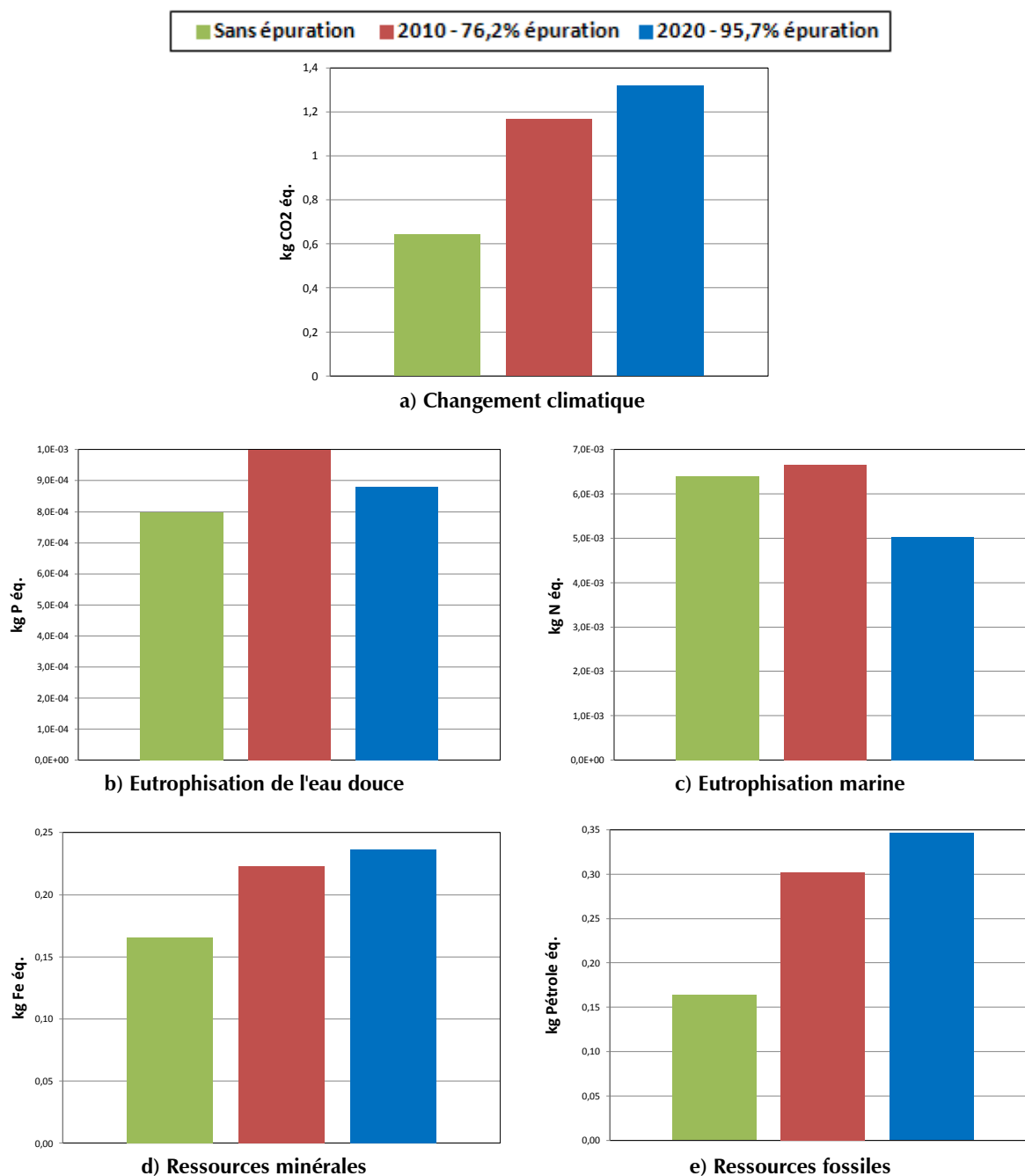
Figure 9: Caractérisation – Comparaisons par catégorie d'impact de différents scénarios selon le taux d'équipement épuratoire pour 1 UF (1m³ d'eau chez l'utilisateur)- ReCiPe Midpoint
