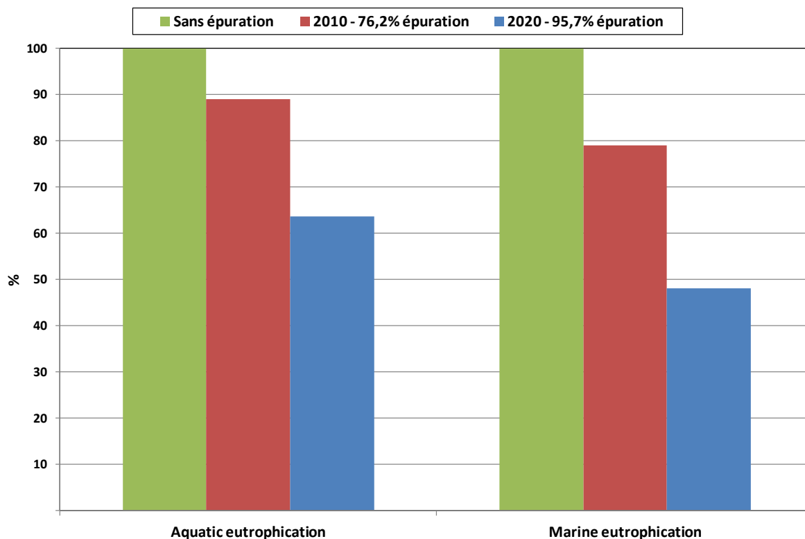
Figure 10: Caractérisation – Comparaisons pour la catégorie de l'eutrophisation de différents scénarios selon le taux d'équipement épuratoire pour 1 UF (1m 3 d'eau chez l'utilisateur) - IMPACT World+ Midpoint
