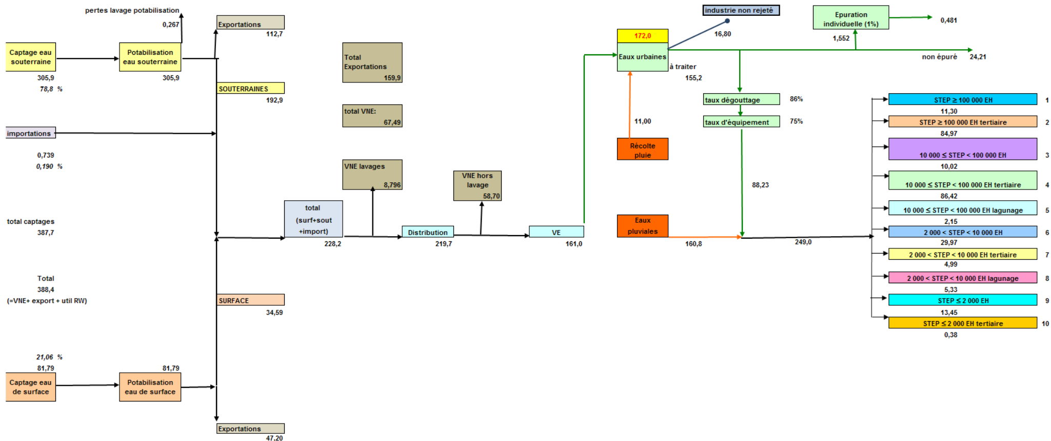
Figure 4: Représentation schématique des flux d'eau de distribution et d'eau de pluie en Région wallonne en millions de m³ – scénario 2010
