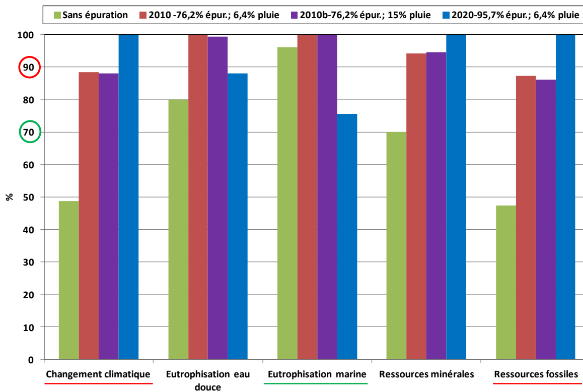
Figure 8: Caractérisation – Comparaison de différents scénarios selon la quantité d'eau de pluie collectée et le taux d'équipement épuratoire pour 1 UF (1m 3 d'eau chez l'utilisateur) - ReCiPe Midpoint
