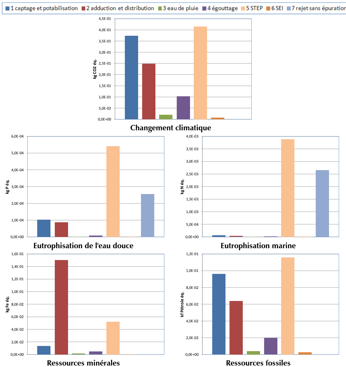
Figure 6: Comparaison par catégorie d'impact des valeurs de caractérisations pour les étapes du cycle anthropique de l'eau pour 1 UF (1m 3 d'eau chez l'utilisateur) – ReCiPe Midpoint
