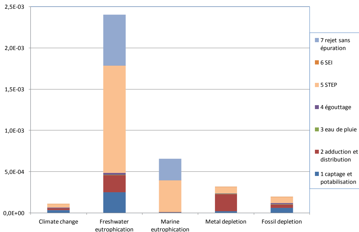
Figure 7: Normalisation cycle global 2010 pour 1 UF (1m 3 d'eau chez l'utilisateur)- ReCiPe Midpoint
